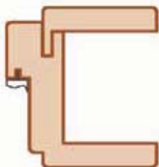
ZB/MB70: muurdikte 70 mm
